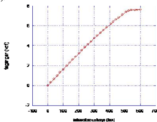
Gambar 1. Grafik hubungan antara lux dengan volt.
