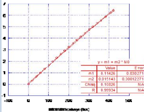
Gambar 2. Grafik kalibrasi fotodiode dengan luxmeter .
