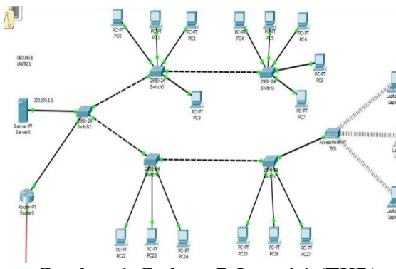
Gambar 6. Gedung B Lantai 1 (TKR)
