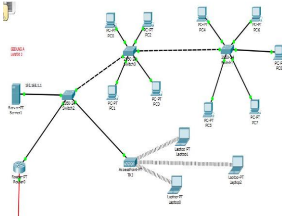
Gambar 4. Gedung A Lantai 1 (TKJ)
